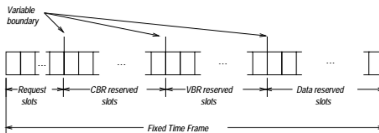
Fig. 1.6 PRMA/DA protocol.
