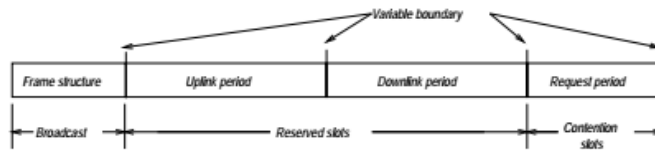
Fig. 1.8 MASCARA protocol.
