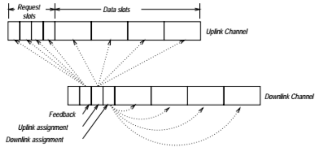
Fig. 1.7 DSA++ protocol.
