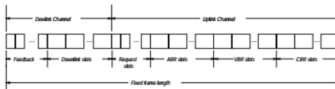
Fig. 1.9 DTDMA protocol.
