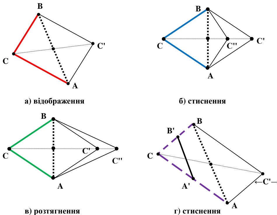
Рис. 5.1. Графічна ілюстрація прийомів симплекс методу Нелдера-Міда
